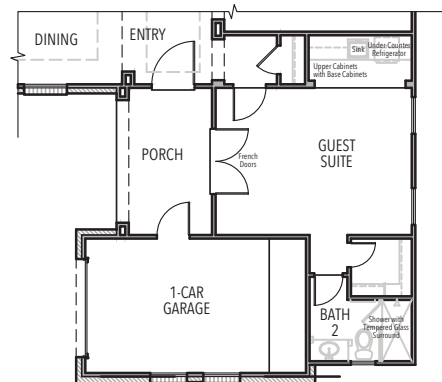
OPTIONAL GUEST SUITE
